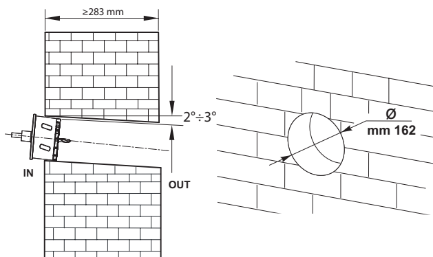
VORT HRW 40/60 MONO EVO - MONTAGE DES GITTERS VON INNEN
