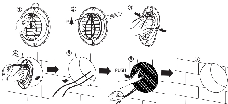
VORT HRW 40/60 MONO EVO - MONTAJE REJILLA DESDE EL EXTERIOR
