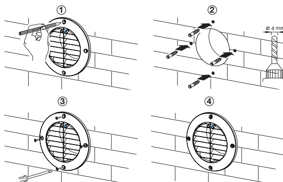
VORT HRW 40/60 MONO EVO - MONTAGE DES GITTERS VON AUSSEN
