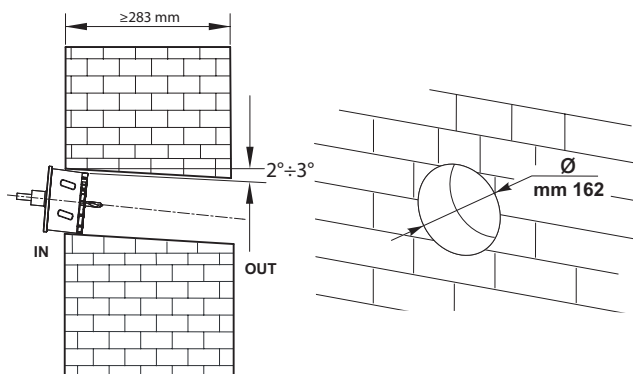
VORT HRW 40/60 MONO EVO - MONTAJE REJILLA DESDE EL INTERIOR
