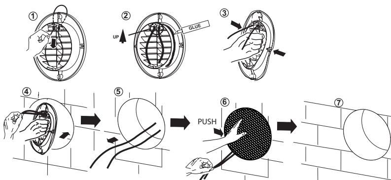
VORT HRW 40/60 MONO EVO - MONTAGE DES GITTERS VON AUSSEN
