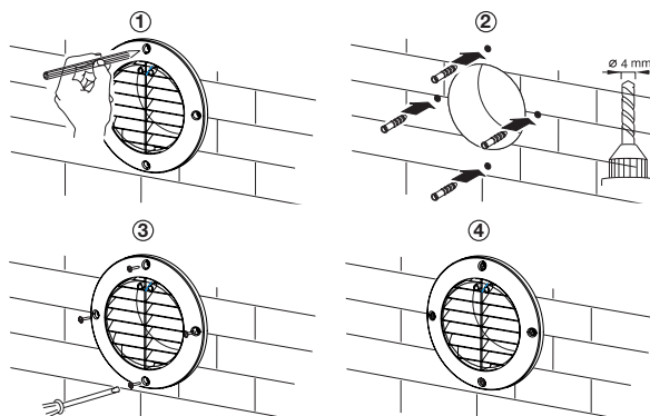
VORT HRW 40/60 MONO EVO - MONTAJE REJILLA DESDE EL EXTERIOR
